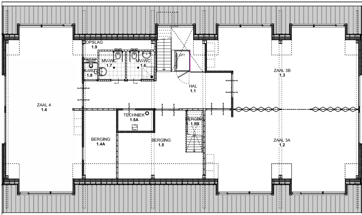
Bouwtekening van de eerste verdieping
