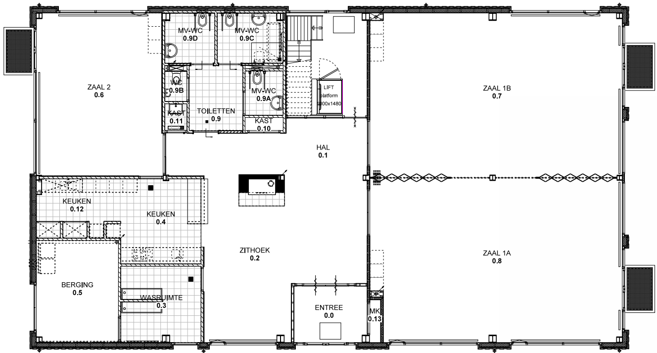
Bouwtekening van de begane grond
